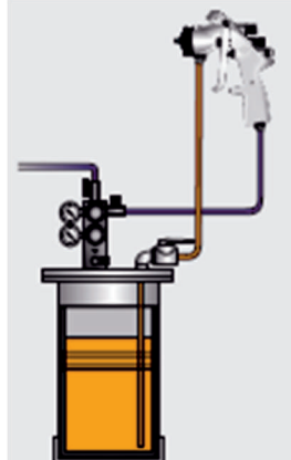
BASINÇLI / BASINÇSIZ KAZANLAR
